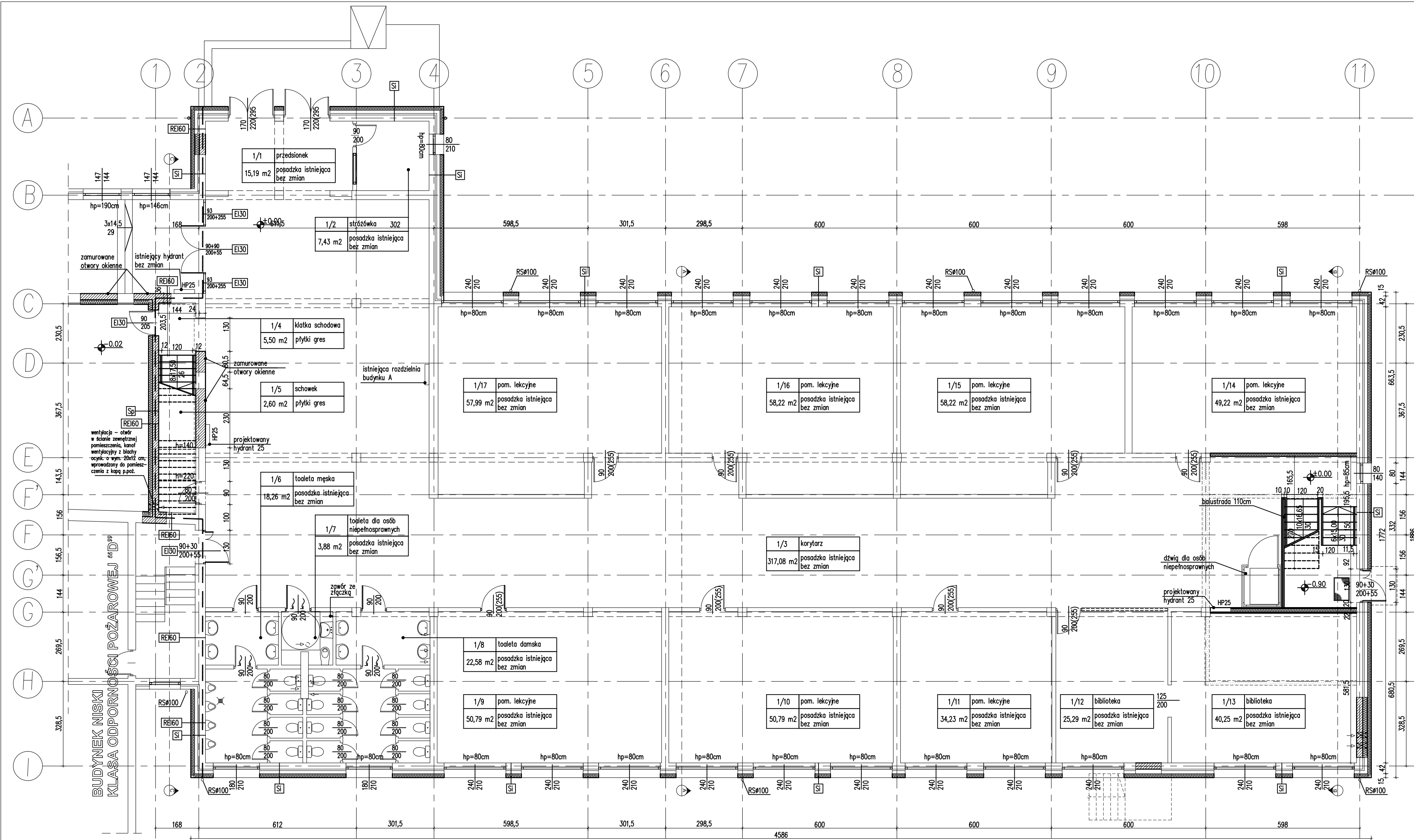
ZESTAWIENIE POWIERZCHNI PARTERU
