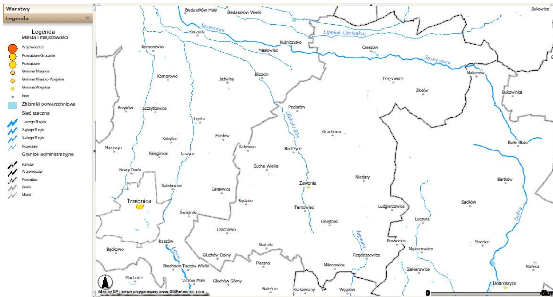
Rysunek 2.22 Sieć hydrograficzna na obszarze gminy [opracowanie własne na podstawie źródła: 33]
