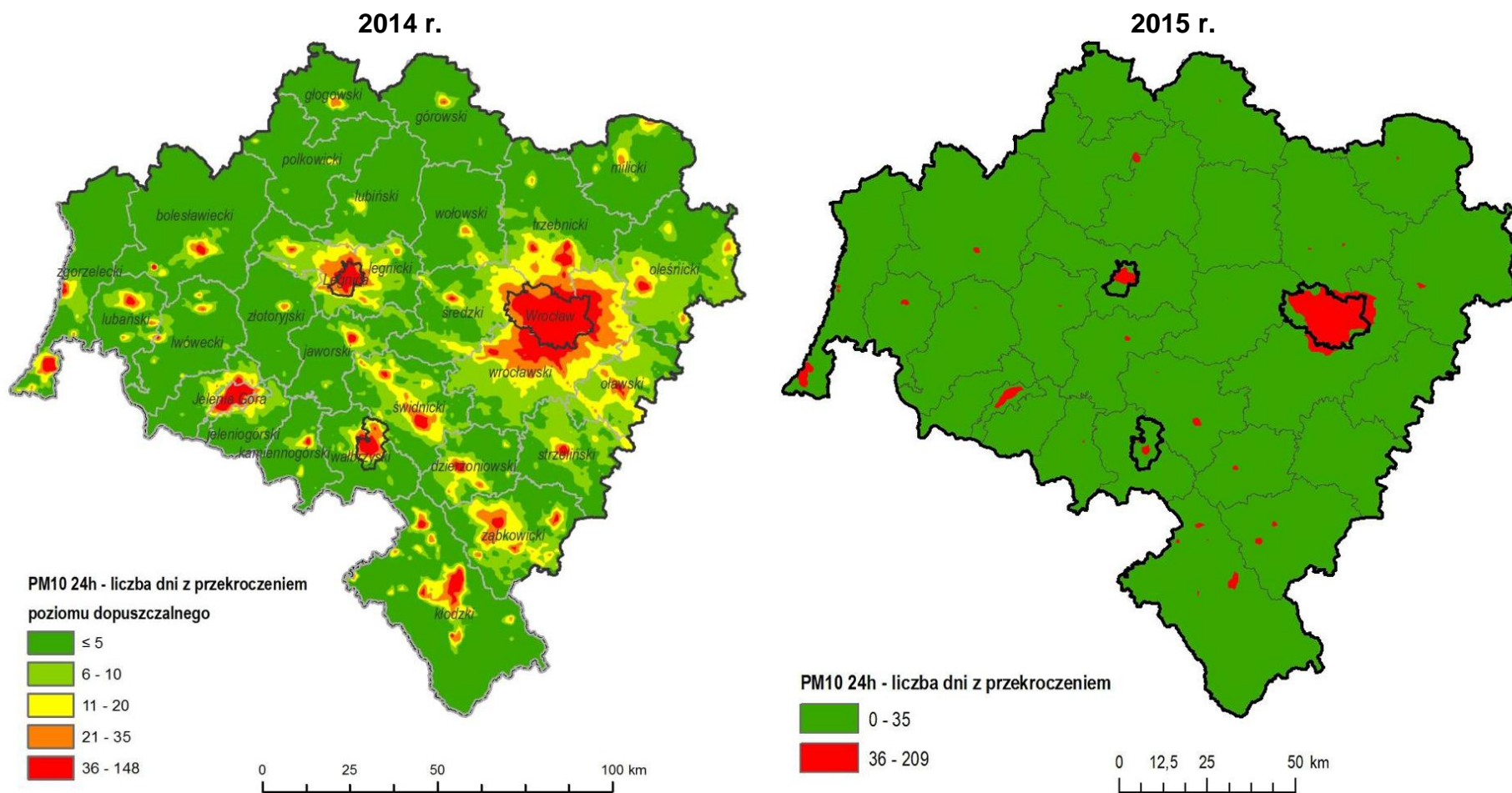
Rysunek 2.12 Rozkłady liczby dni z przekroczeniami dopuszczalnego poziomu 24-godzinnego pyłu zawieszonego PM10 na terenie województwa dolnośląskiego na podstawie wyników modelowania jakości powietrza opracowanych przez WIOŚ we Wrocławiu za 2014 i 2015 r. [25, 26]
